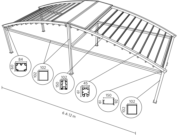
GAZEBO DE DUAS ÁGUAS DUPLO
